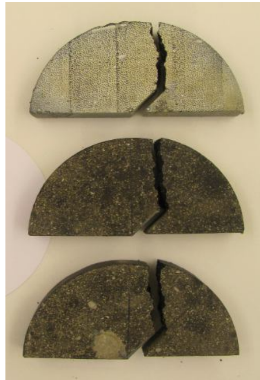
(4) 45°, s/r=0.8
